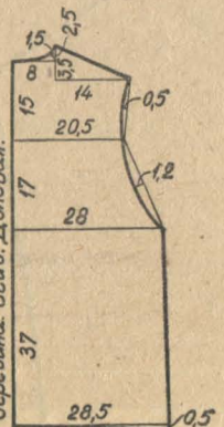
Спинка жилета 1 дет.
