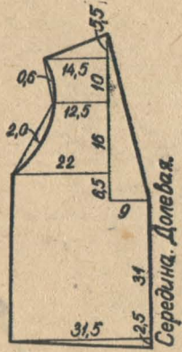
Полочка жилета 2 дет.
